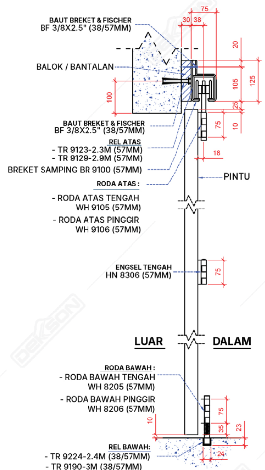
Gambar Potongan
