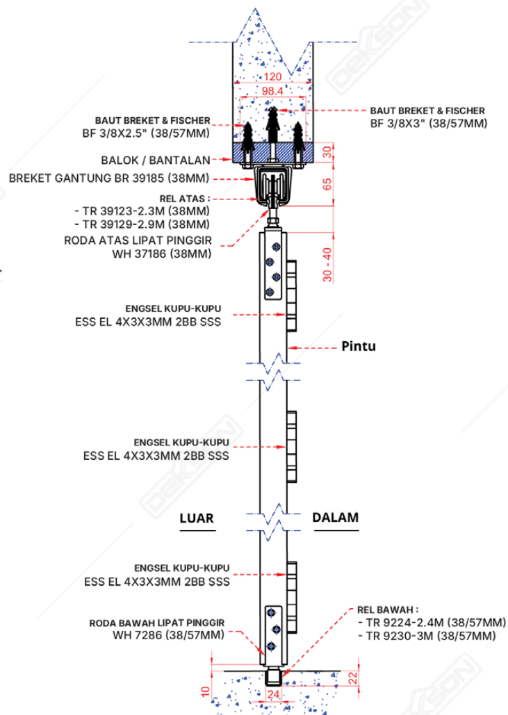
Gambar Potongan
