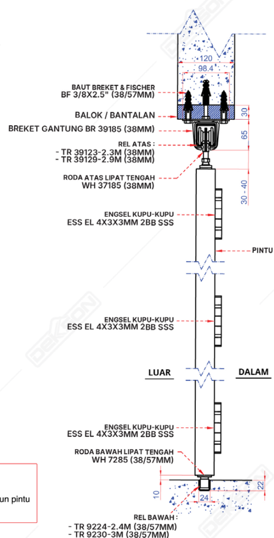
Gambar Potongan
