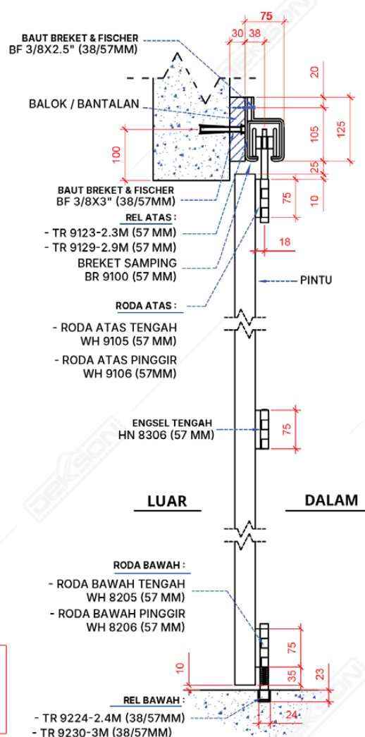
Gambar Potongan
