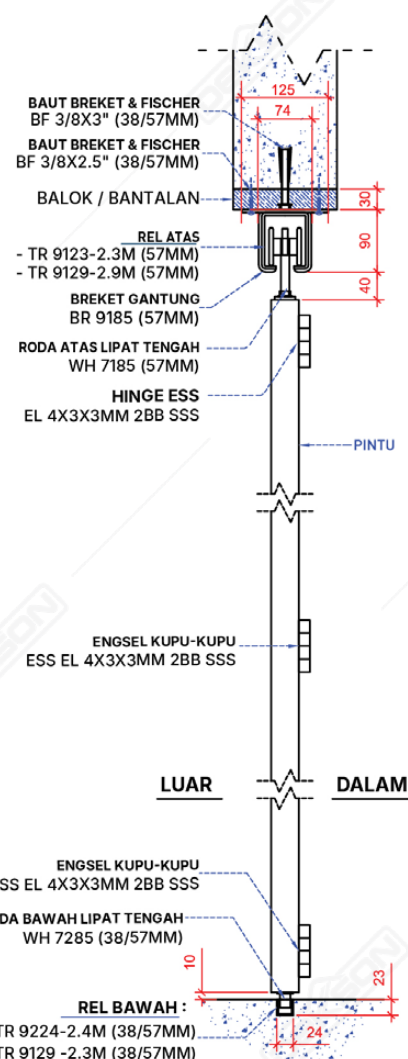
Gambar Potongan
