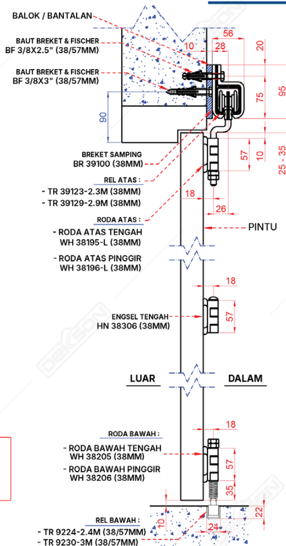
Gambar Potongan
