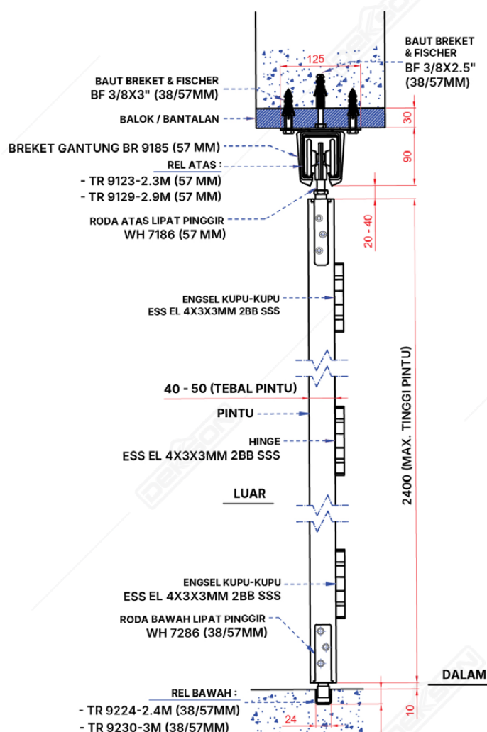
Gambar Potongan
